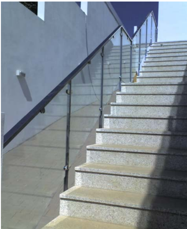
Pasamanos con estructura de acero y vidrio laminado de seguridad, fijado con pinzas también de acero
